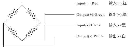
Wiring Diagram/接线图
